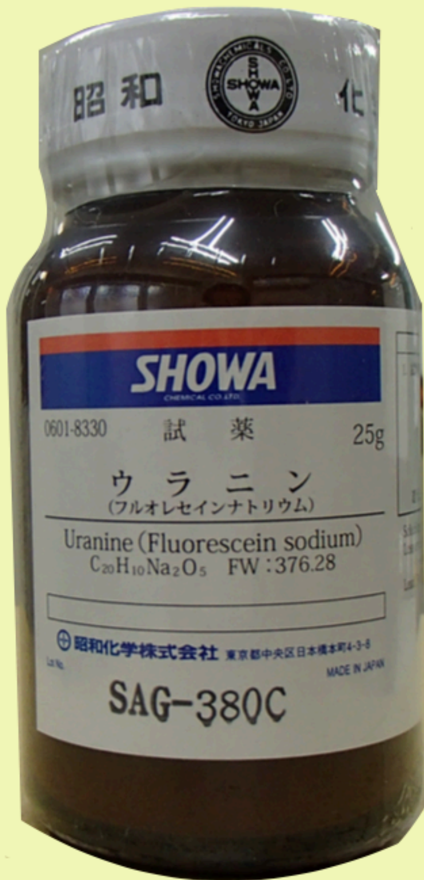
ウラニン (フルオレセインナトリウム)
