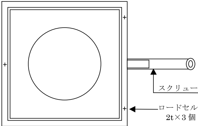
上面図
